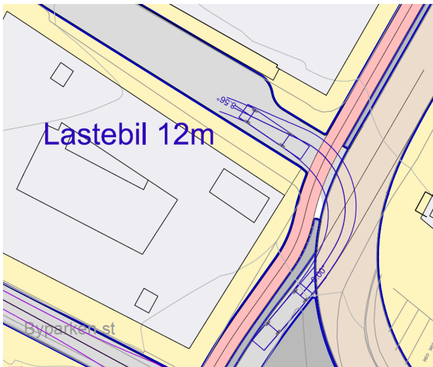
Figur 4.2-2 Skisse som viser sporingskurve for 12 m lastebil fra Christies gate til Rådhusgaten. Resulterende fall mot påkobling i Christies gate/ banetrasé kan bli under 2 %, eventuelt behov for fravik avklares i byggeplanfase.
