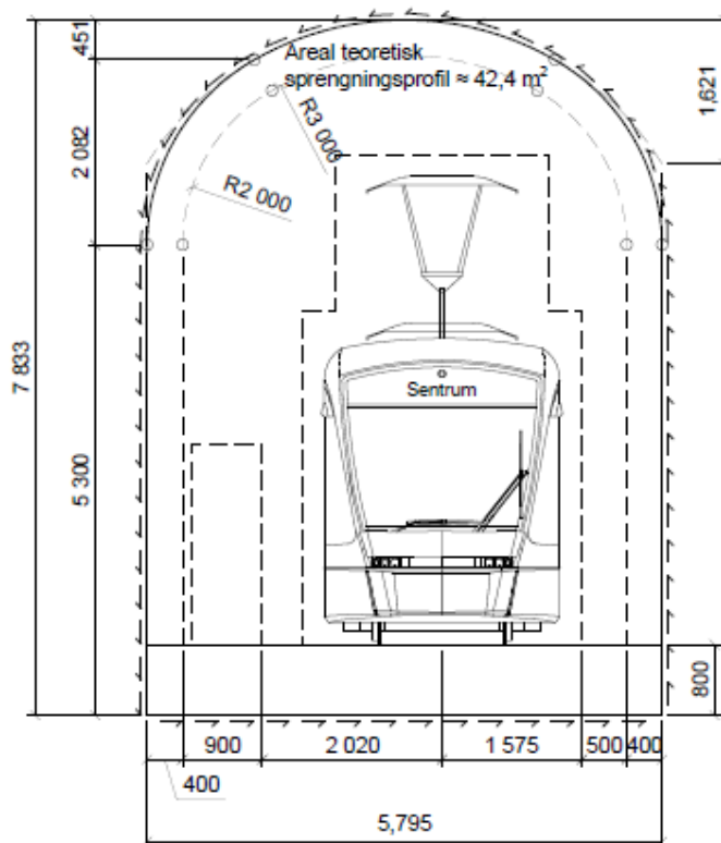
Figur 3.5-3 Tverrsnitt ettsportunnel
