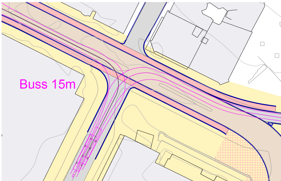
Figur 4.2-3 Skisse som viser sporingskurver for 15 m buss fra Småstrandgaten til Olav Kyrres gate.
