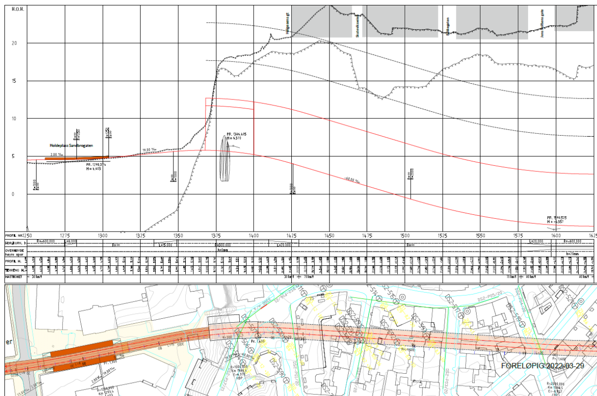
Figur 3.1-9: Oversikt anbefalt bybanetrase med jernbanetunnel på tvers av bybaneportal
