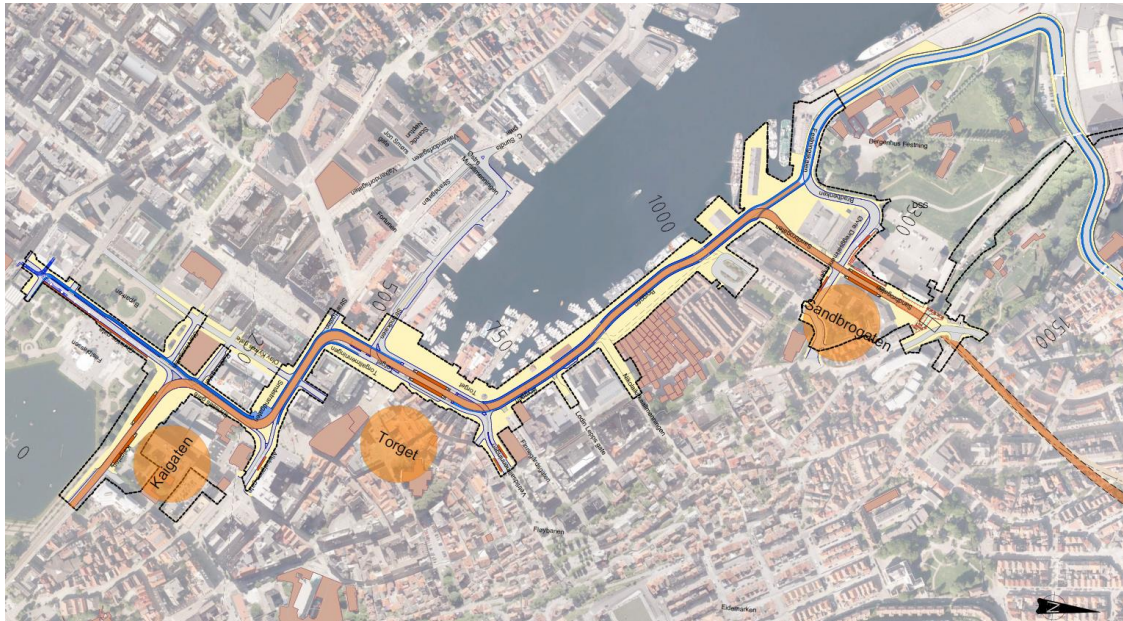
Figur 4.1.3.5-1 Utklipp av oversiktsplan (B-tegning) som viser løsningen.
