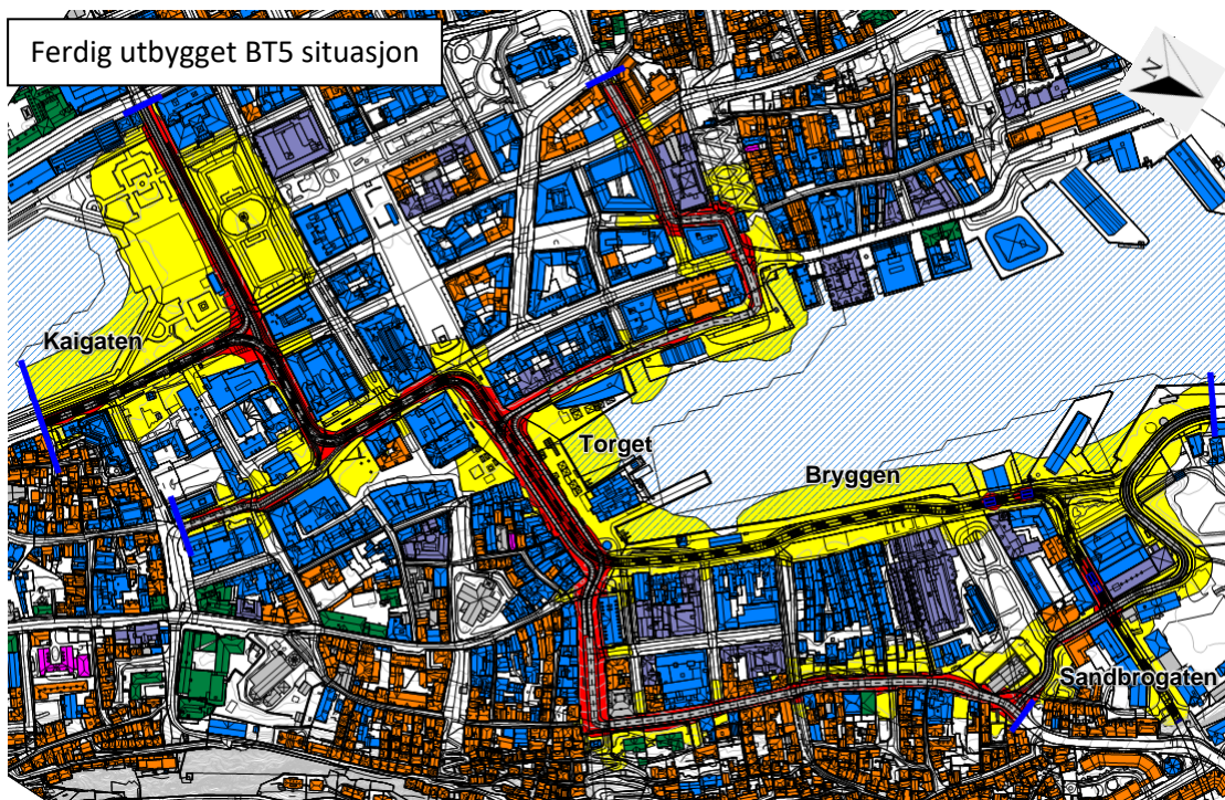
Figur 4.7-3 Samlet støynivå fra veg og bane i ferdig utbygget BT5 situasjon beregnet 4 m.o.t. Gul støysone, L_{den} > 55 dB, rød støysone L_{den} > 65 dB. Nord er ned til høyre i figuren.
