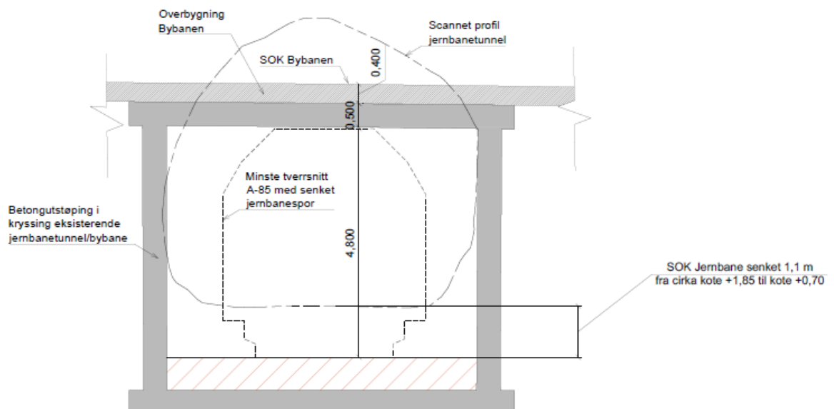
Figur 3.1-11: Prinsippsnitt som viser hvordan bybanespolet vil krysse jernbanetunnelen
