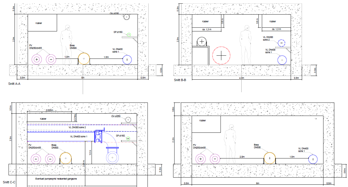
Figur 4.4-1 Prinsippnitt VA-kulvert, Harbitzthjørnet
