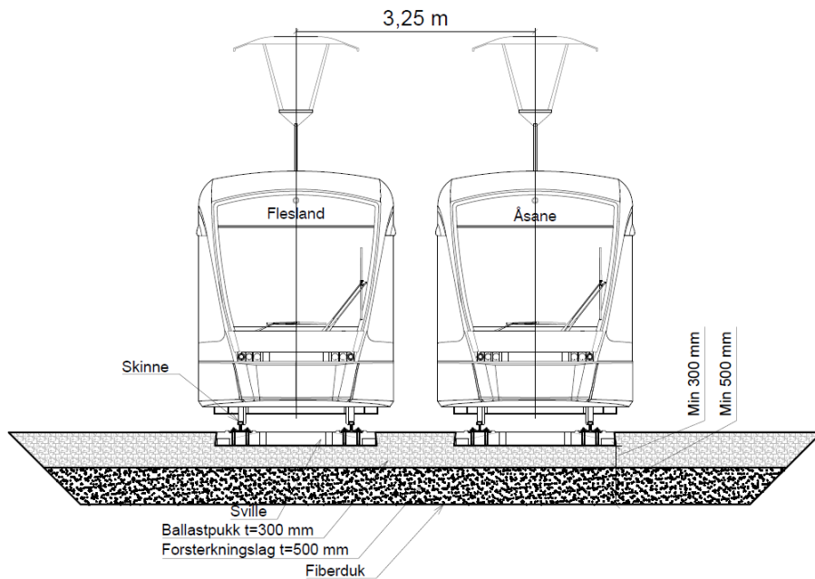
Figur 7.3-1 Normalprofil bane, ballastspor
