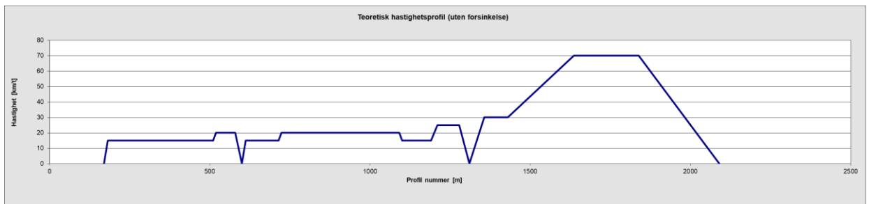
Figur 3.1-1: Hastighetsprofil DS1.
