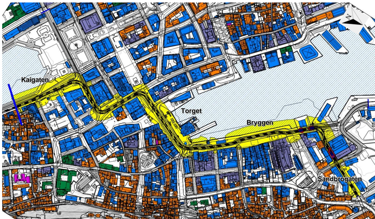
Figur 4.7-2 Støyutbredelse av gul støysone ( L_{den} > 58 dB) og rød støysone ( L_{den} > 68 dB) fra bane i ferdig utbygget BT5 situasjon beregnet 4 m.o.t. Nord er ned til høyre i figuren.
