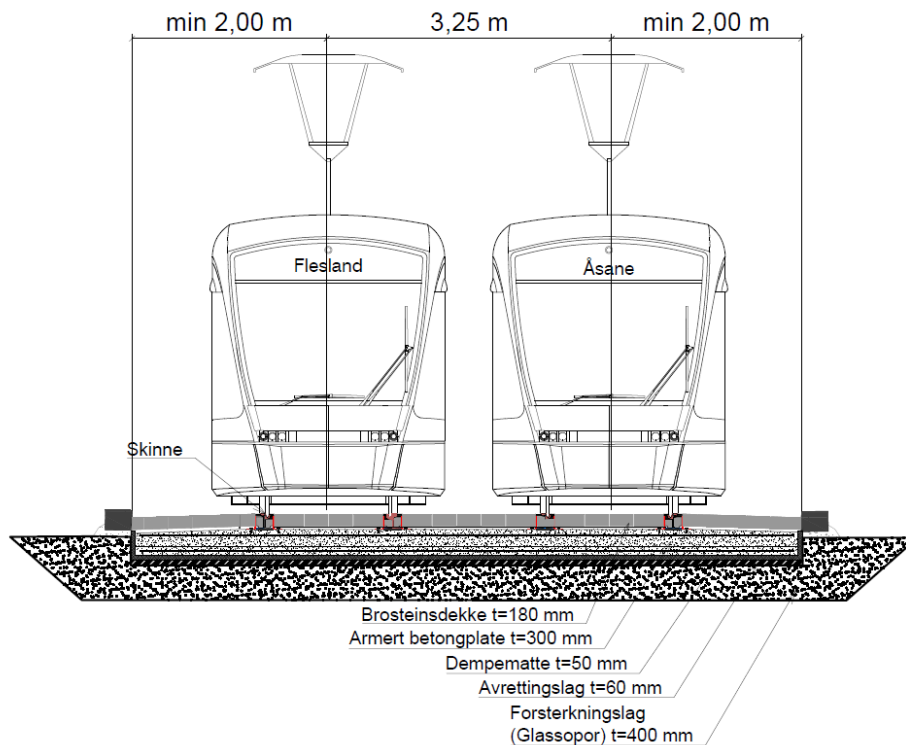
Figur 2.2-2 Prinsippkisse for oppbygging av banetrase med Glasopor ned mot undergrunnen og under betongplaten for banesporet. Platefundamentet sin bredde kan velges for å påvirke løsningen for å oppnå lav, midlere tilleggslast på undergrunnen.
