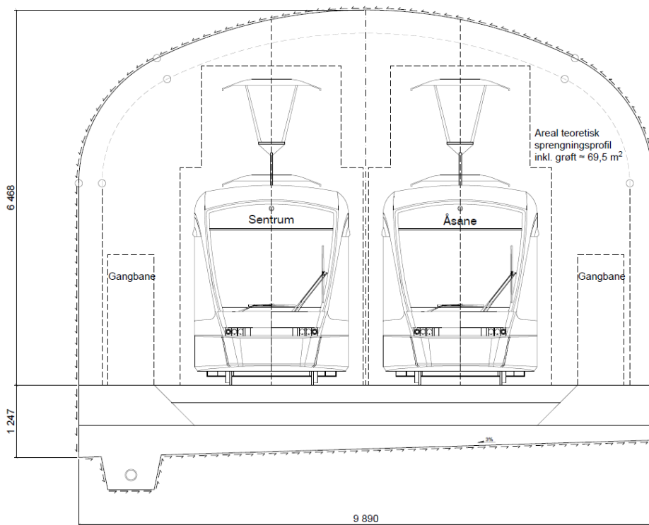
Figur 3.5-2 Tverrsnitt dobbeltsportunnel
