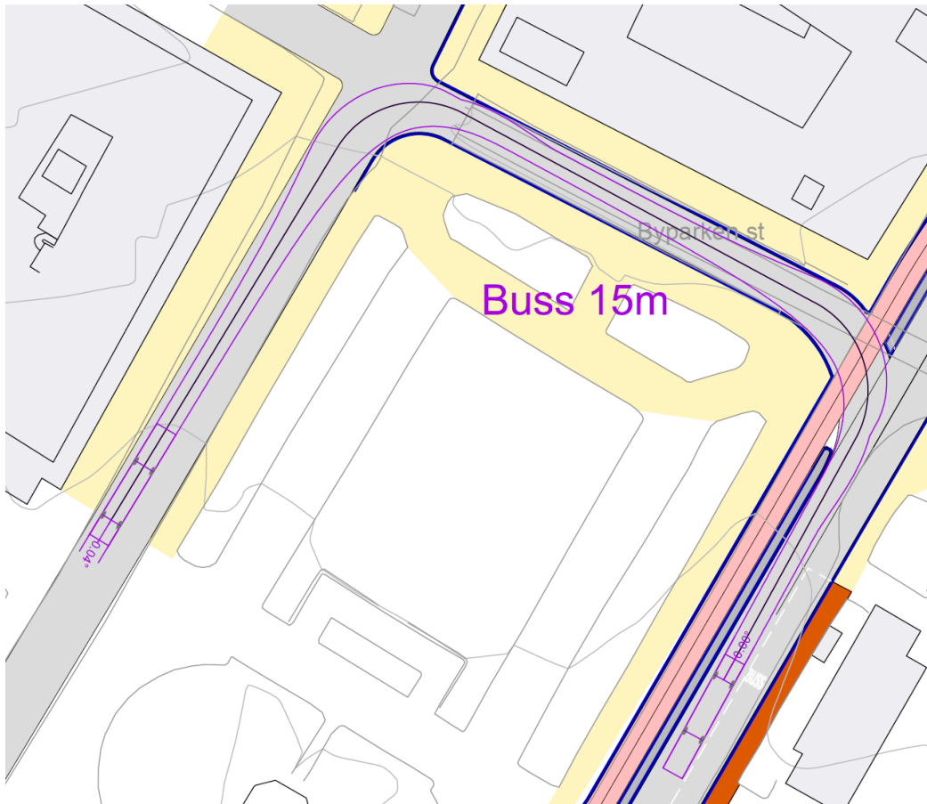
Figur 4.2-1 Skisse som viser sporingskurve for 15 m buss fra Christies gate gjennom Starvhusgaten til Olav Kyrres gate.
